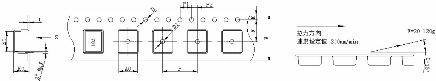
载带尺寸 (TAPE DIMENSIONS) 一般公差为±0.1mm
