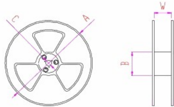
卷轴尺寸 (REEL DIMENSIONS) 一般公差为±0.5mm
