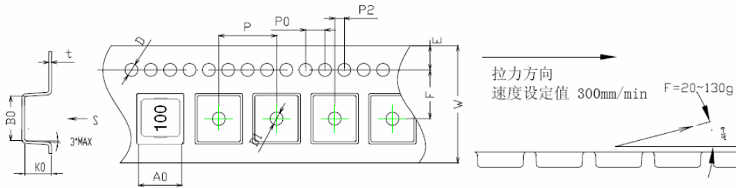
载带尺寸 (TAPE DIMENSIONS) 一般公差为±0.1mm
