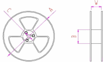
卷轴尺寸 (REEL DIMENSIONS) 一般公差为±0.5mm
